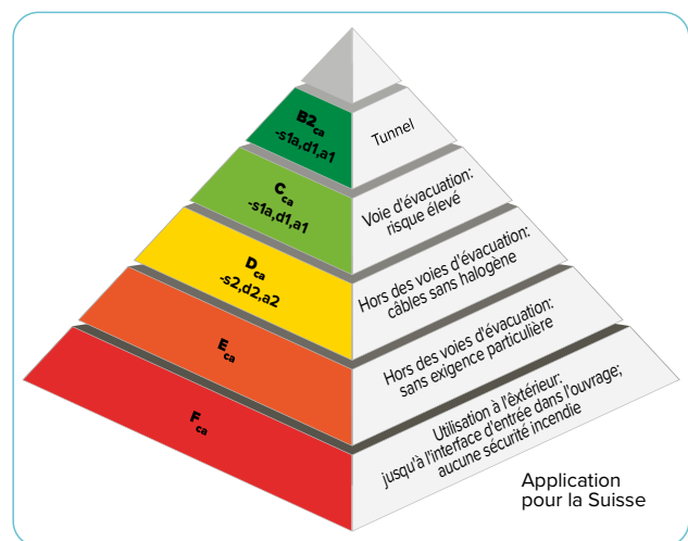
Les propriétés sont testées selon l'OPCo, avec classification B2 ca -s1a,d1,a1
