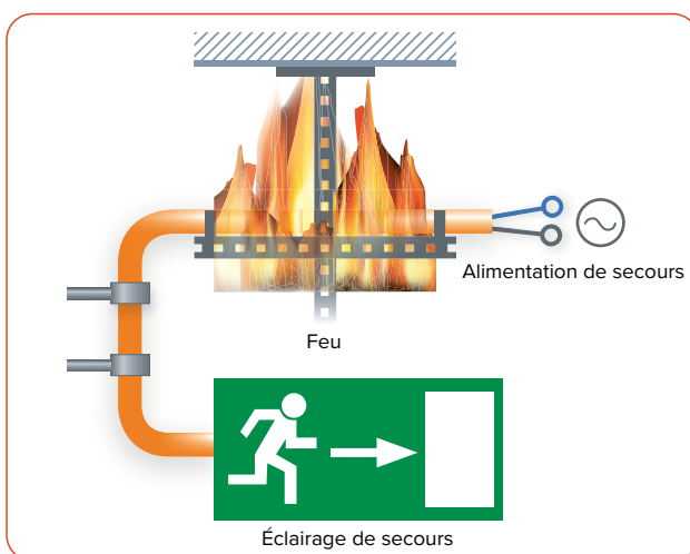
Le câble et le chemin de câble sont testés ensemble lors de la simulation d'un grand incendie (four).
